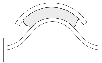
Fissaggio coppi con malta magra di cemento Fig. 26a
