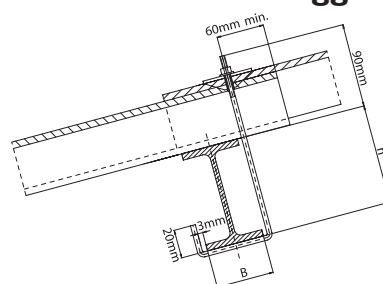
gancio L su trave IPE Fig. 21b
