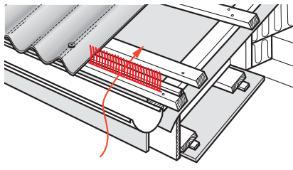
Griglia parapasseri Fig. 14b
