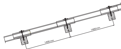
Interasse di appoggio 1400 mm Fig. 11b
