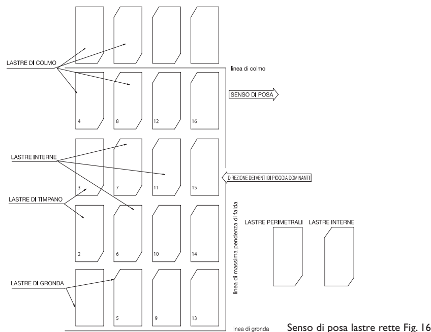
Senso di posa lastre rette Fig. 16
