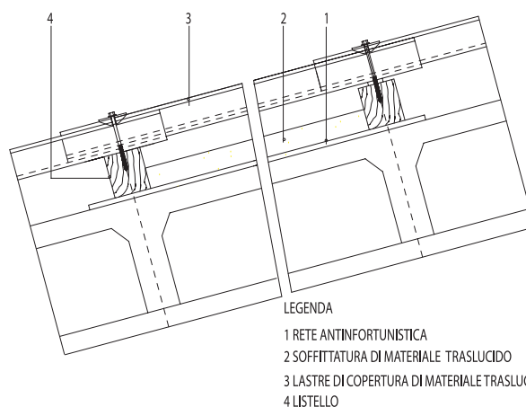
sicurezza nei cantieri Fig. 33b
