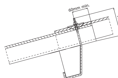
gancio sagomato su c.a Fig. 21f
