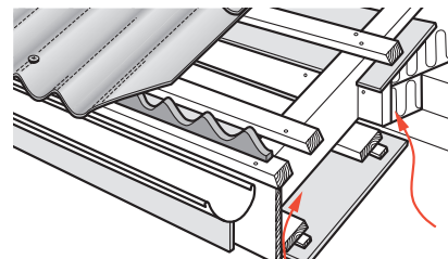
Interspazi di ventilazione nelle gronde Fig. 14c
