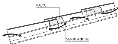
Fissaggio coppi con malta magra di cemento esempio ventilazione Fig. 26b
