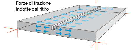
Frattura massetto con sfogo della tensione da ritiro nel giunto preimpostato
