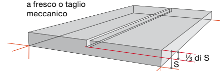
Forze di trazione indotte dal ritiro
